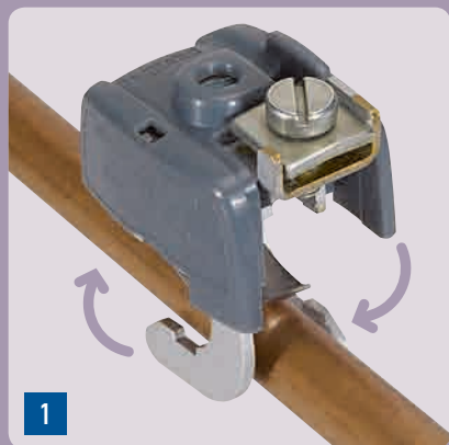
1 Engagemment par pression sur le tube et fixation par 1/4 de tour
